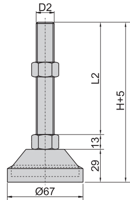
KMS60 配加防滑橡膠盤墊
