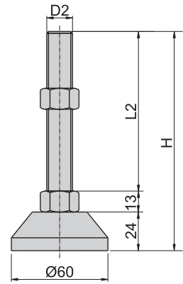
S60 無防滑橡膠盤墊
