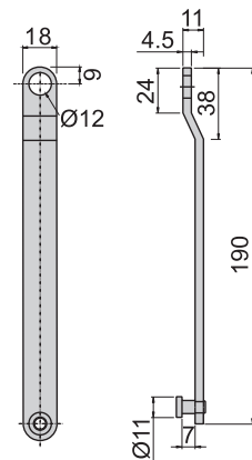
B-1083-S4 B-83-S4
