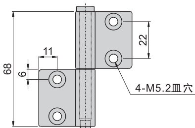
1702#、702# 用心軸
