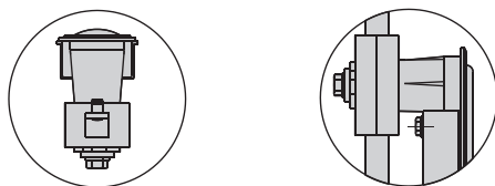
把手附天地栓結構示範圍
