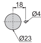
逆時針開孔尺寸圖
