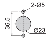
順時針開孔尺寸圖
