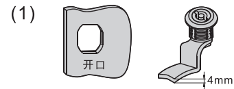
可先裝配直角回轉鎖
