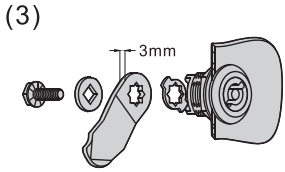
方向與與角度配合擋件片組方法
