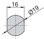
開孔尺寸圖
